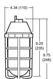
Pendant Incandescent
