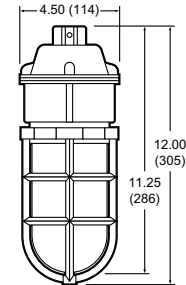
Pendant Fluorescent, HID
