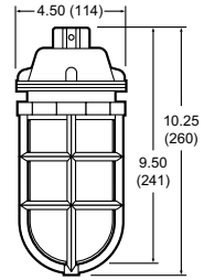
Pendant Incandescent
